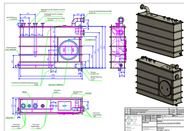
Beispiel 3D-Zeichnung Spülwasserbehälter
