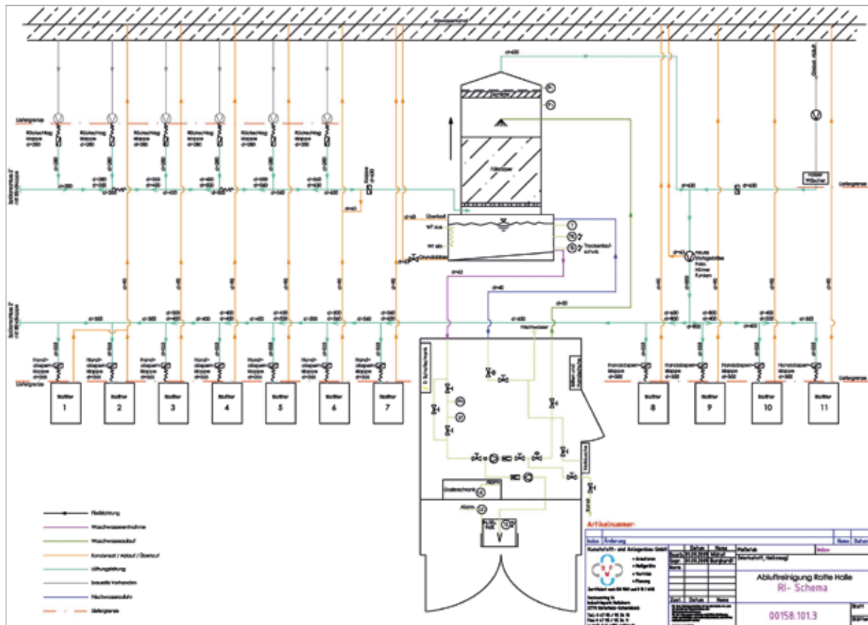
Beispiel Abluftreinigung RI-Schema
