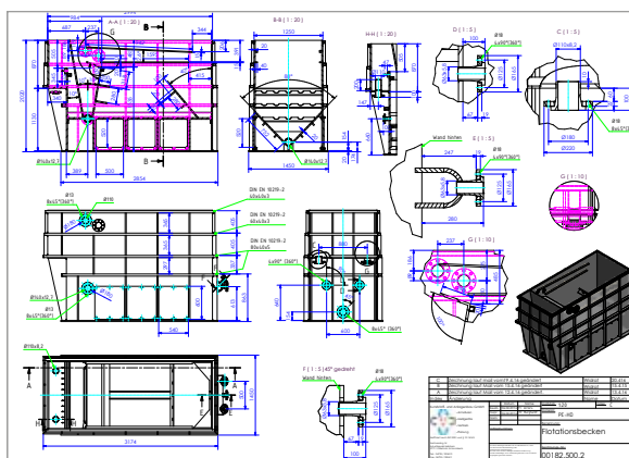
Beispiel 3D-Zeichnung Flotationsbecken
