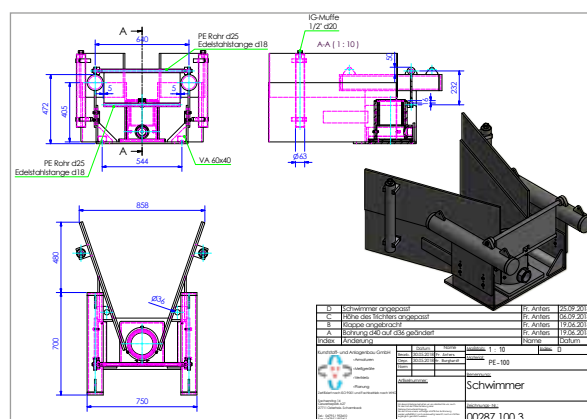
Beispiel 3D-Zeichnung Schwimmer
